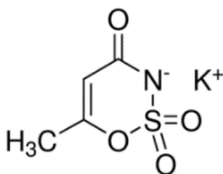
Figura 1: Formula Molecular do Acessulfame-K.
